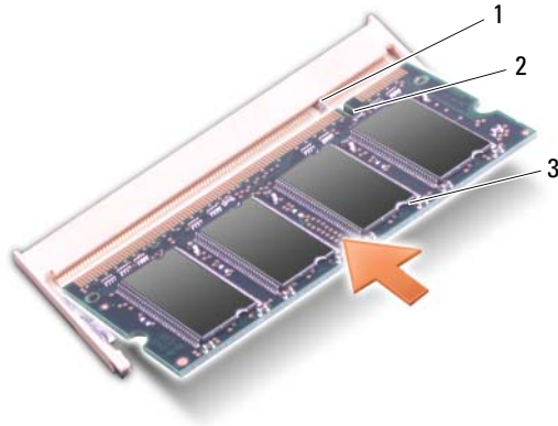
1 彈片 2 槽口 3 記憶體模組
