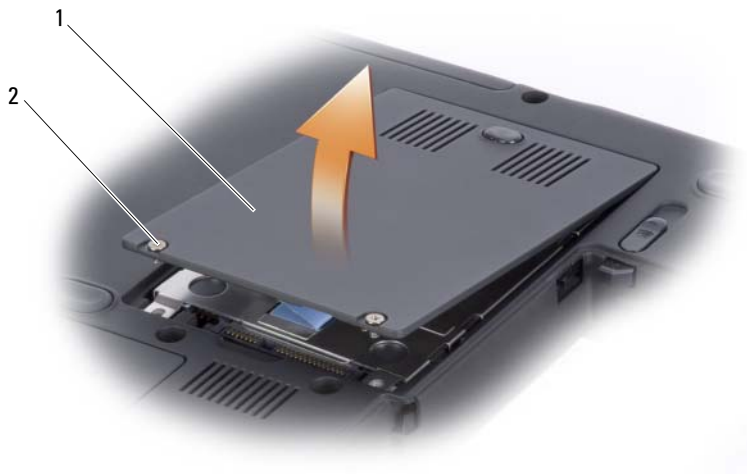
1 硬碟機護蓋 2 螺絲 (2)
