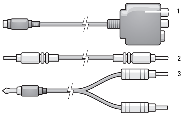
1 合成式影像配接器
